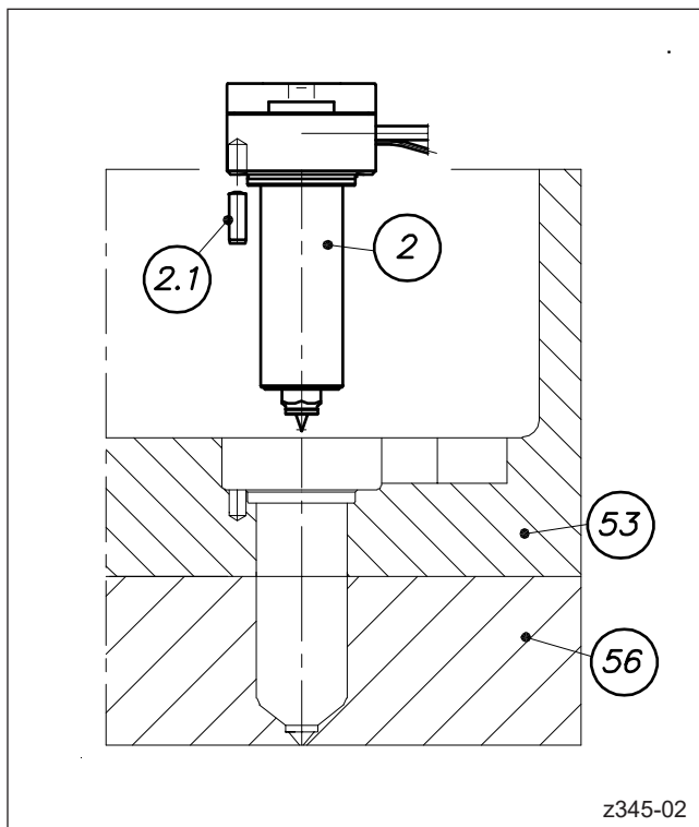
Abbildung 24: Standardmontage einer HPS III-S / pro SHOT Systemdüse
