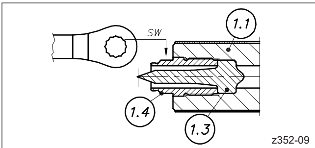
Abbildung 63: Mundstück herausdrahten
