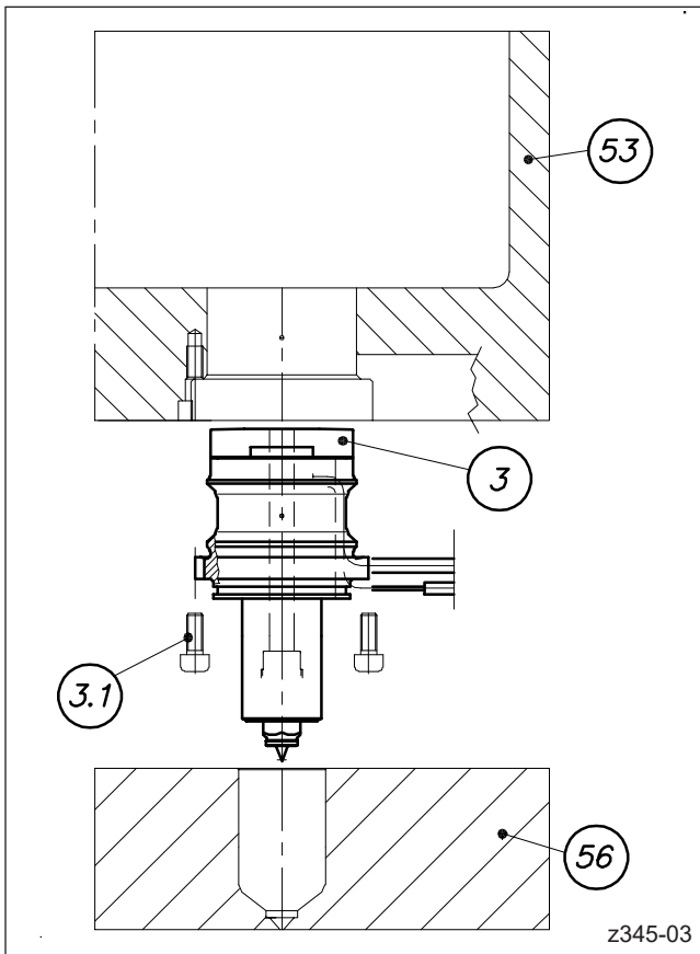
Abbildung 25: Frontmontage einer HPS III-S / pro SHOT Systemdüse
