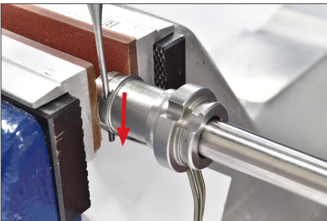
Abbildung 72: Spannhülsen heraus schlagen
