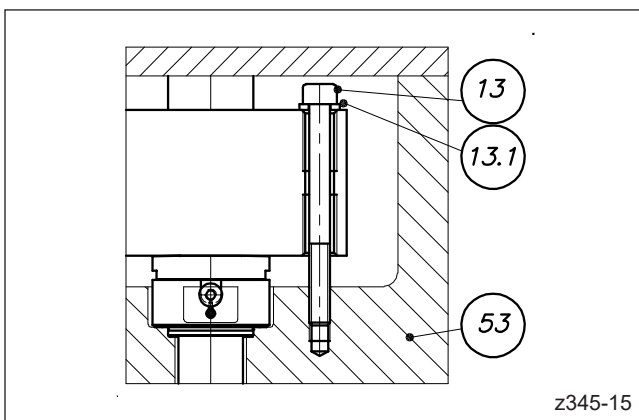
Abbildung 38: Verteilerverschraubung mit Zylinderschrauben (Nur für Standardmontage!)
