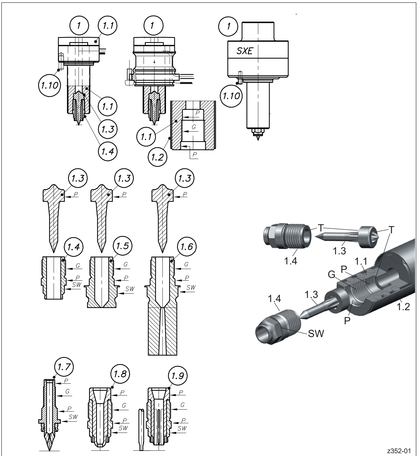
Abbildung 54: Übersicht der verschiedenen Typen von Düsenstipen sowie der zugehörigen Mundstücken und Schraubvorkammern
