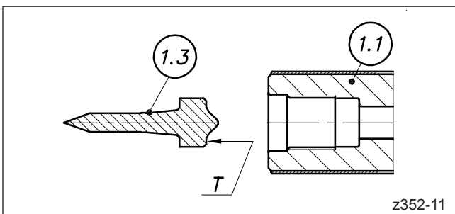
Abbildung 65: Düsenspitze herausziehen
