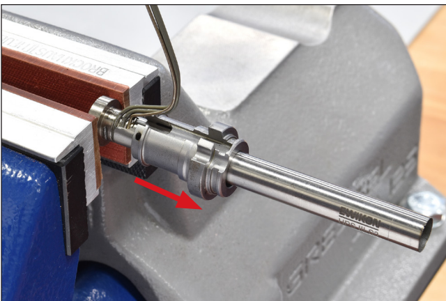
Abbildung 73: Düsenkörper abziehen
