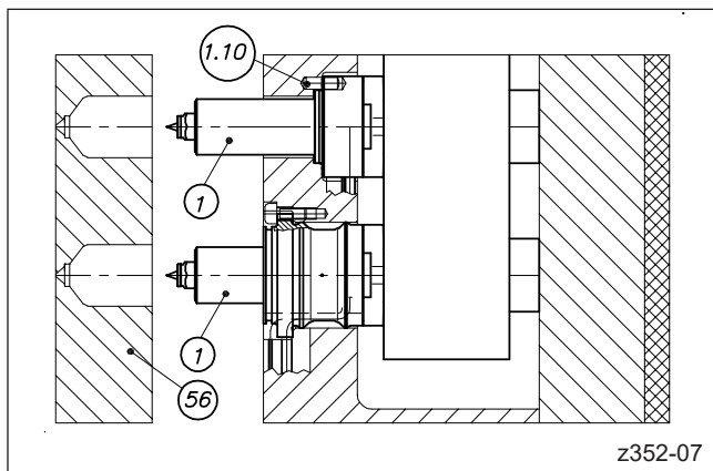
Abbildung 56: Konturplatte entfernen (HPS III-S / pro SHOT Düse)
