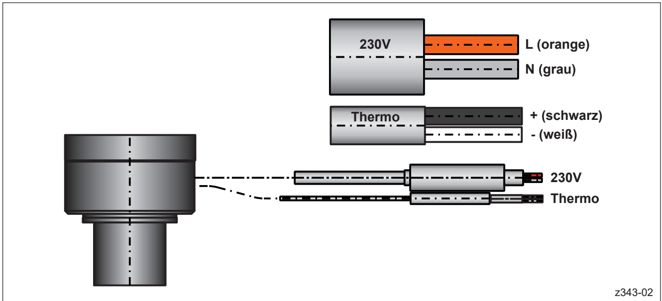
Abbildung 42: Kabelbelegung für HPS III-S / pro SHOT Düsen (ein Regelkreis)
