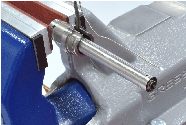
Abbildung 84: Benetzte Fühlerspitze
