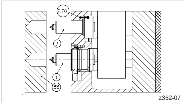
Abbildung 61: Konturplatte entfernen (HPS III-S / pro SHOT Düse)
