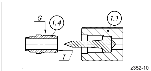
Abbildung 64: Mundstück herausgedrahtet
