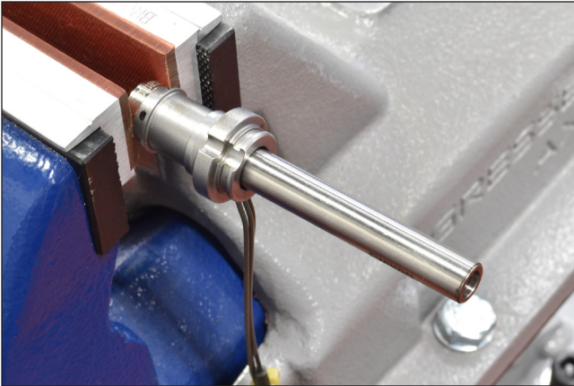
Abbildung 71: Düse einspannen
