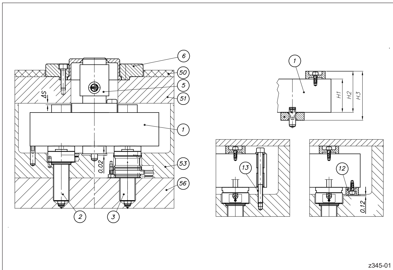
Abbildung 23: Prinzipieller Aufbau eines Systems mit HPS III-S / pro SHOT Düsen für Standard- und Frontmontage
